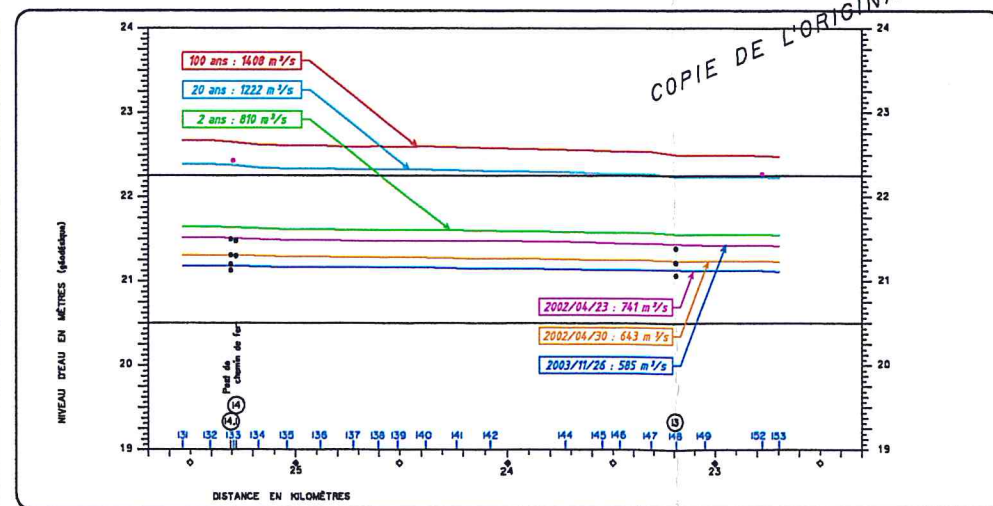
FIGURE 10 PROFIL DES PLANS D'EAU DE LA RIVIÈRE DES MILLE ÎLES SECTEUR DE ROSEMÈRE LÉGENDE : Profil de plan d'eau de récurrence de 100 ans Profil de plan d'eau de récurrence de 20 ans Profil de plan d'eau de récurrence de 2 ans Site de calcul de niveaux d'eau Niveau d'eau observé Niveau théor. par arpentage le 22-05-1974 Site d'observation de niveaux d'eau Distance en kilomètres ÉCHELLE HORIZONTALE : 1 : 20 000 ÉCHELLE VERTICALE : 1 : 50
