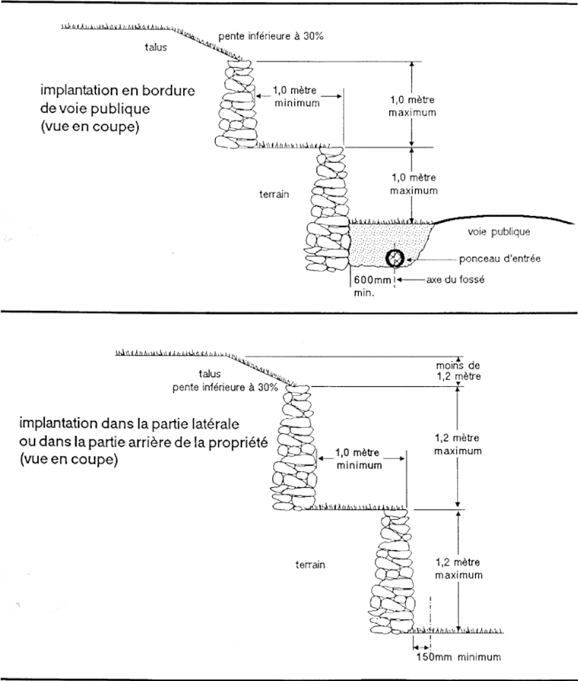
Murs de soutènement et talus illustration
